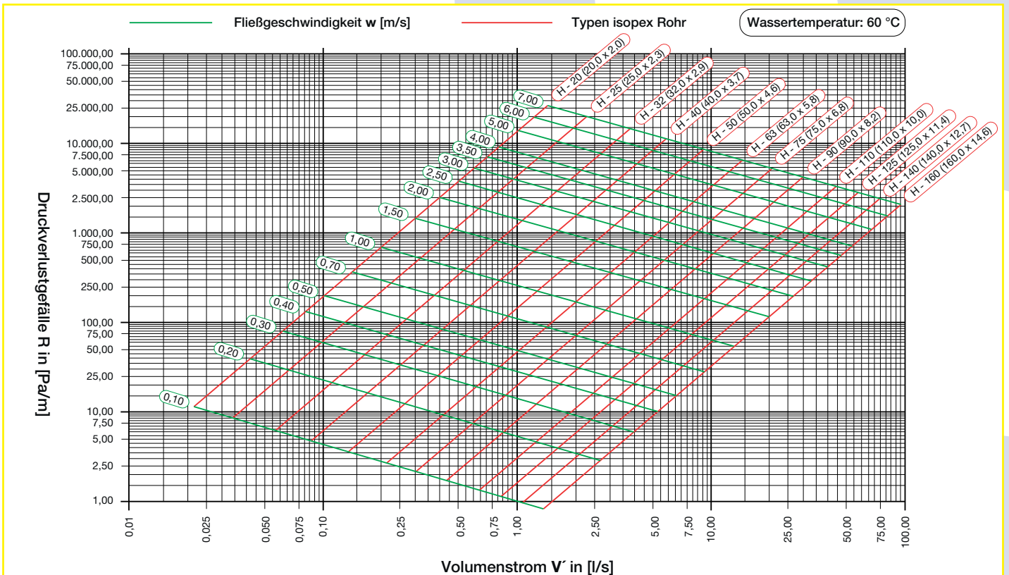
Druckverlustdiagramm SDR 11
